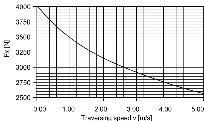
F_x - v - Diagram
